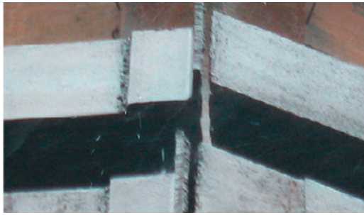
지보공 상부 자재적재 불량II
