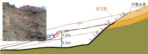
단지조성 시 붕괴
