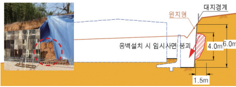
옹벽설치 시 붕괴
