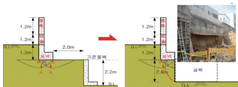
기존옹벽 하부 굴착 시 붕괴
