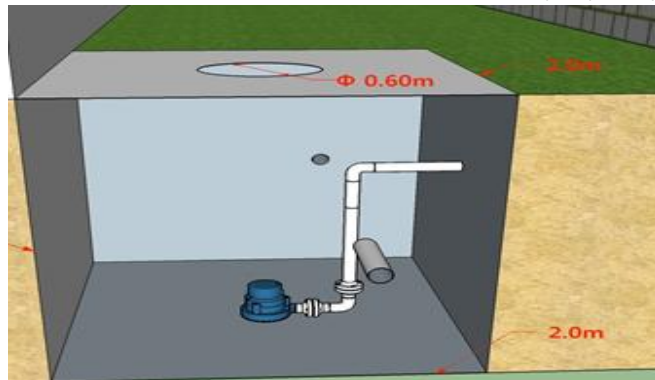
오수집수조 내부 구조도
