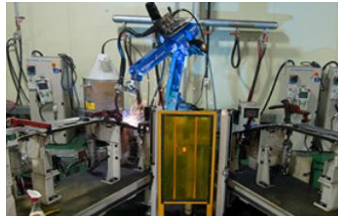
5 로봇 용접작업
