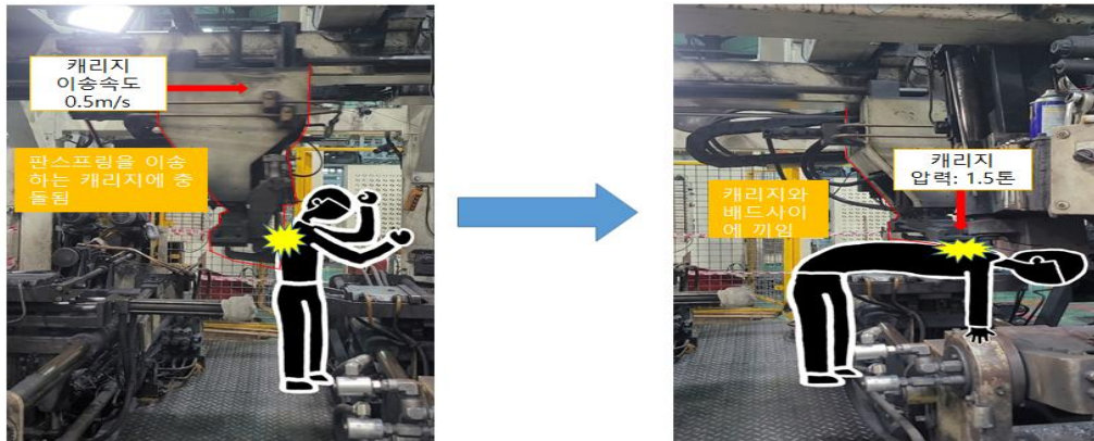
재해발생 상황도
