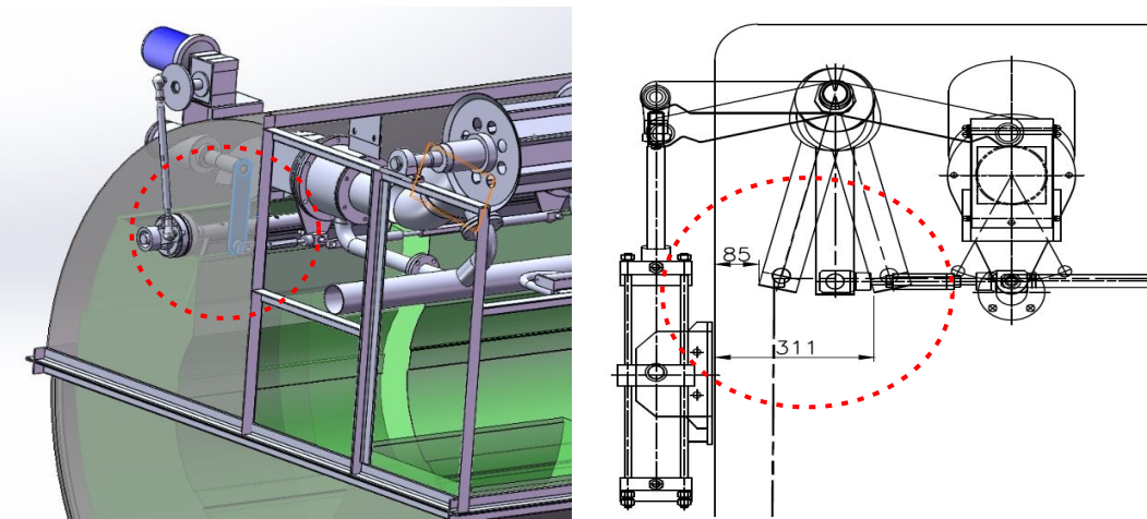
ㄱ자형관-흔들장치 링크부위 모습
