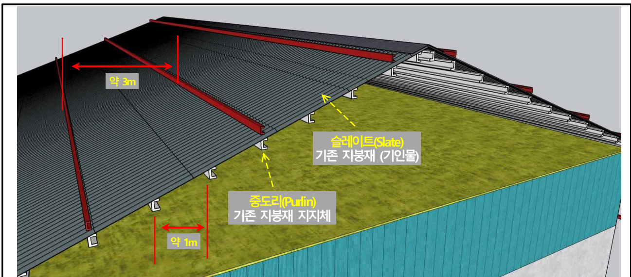
[그림 1] 사고 장소 지붕의 모습 도식화
